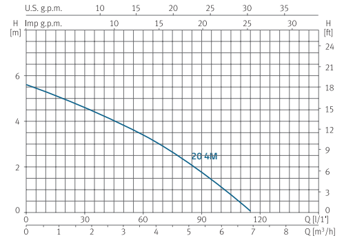
Courbe de fonctionnement à 2900 rpm
