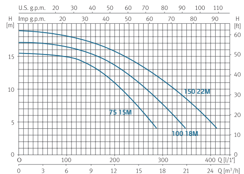
Courbes de fonctionnement à 2900 rpm
