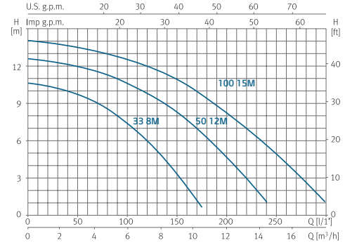
Courbes de fonctionnement à 2900 rpm
